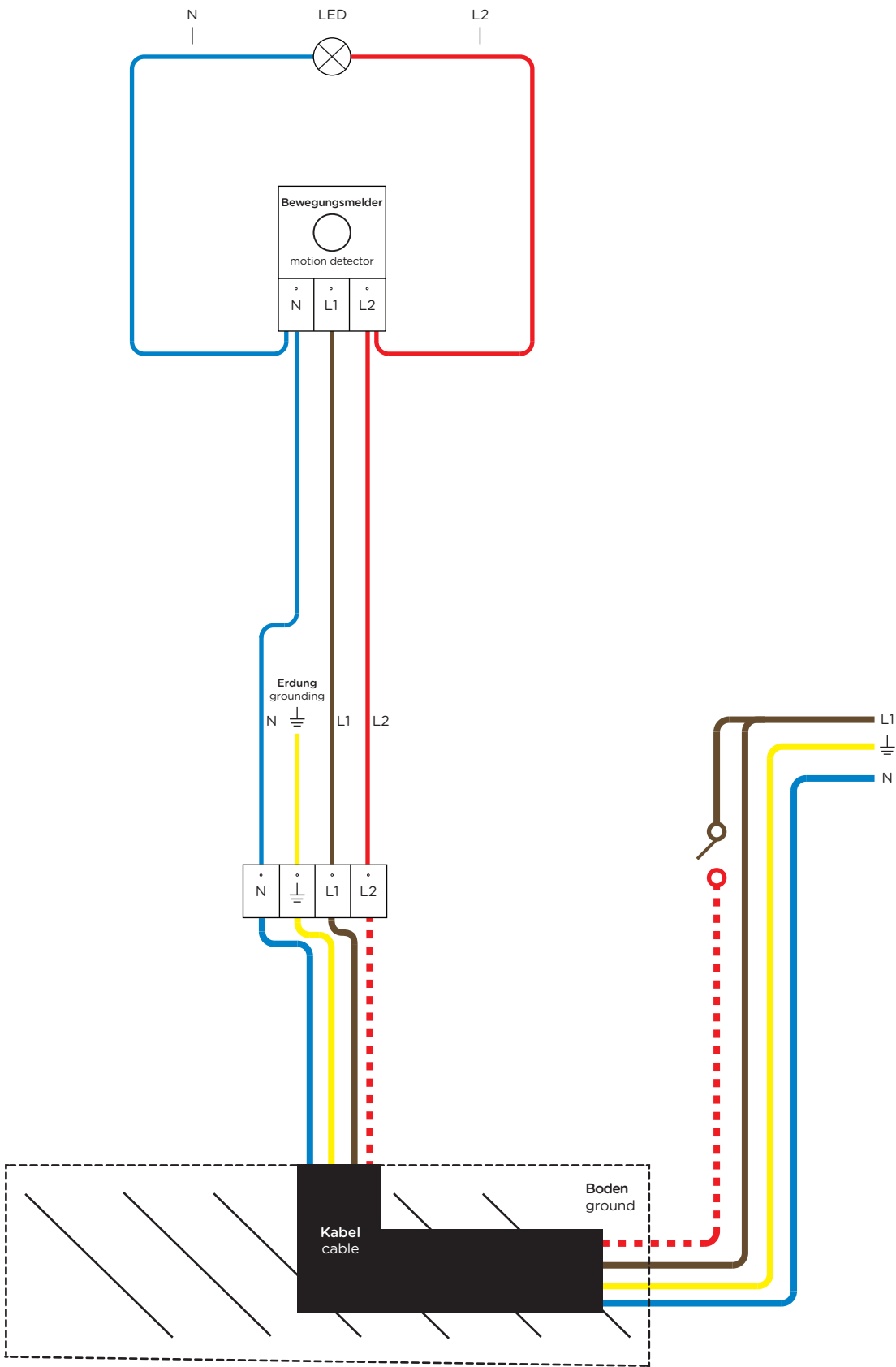
Anschlusschema 4-adrig wiring diagram 4-core
